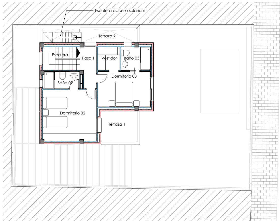
Planta Primera 1 : 150
