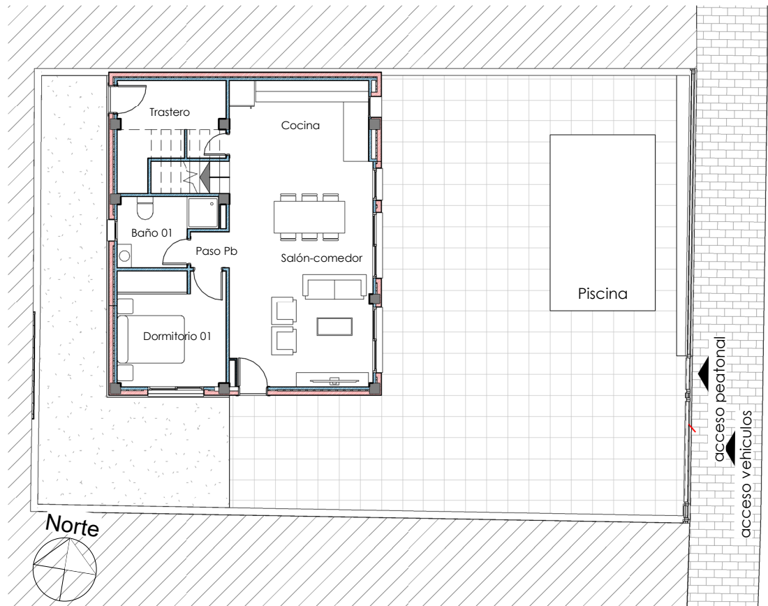
Planta Baja 1 : 150
